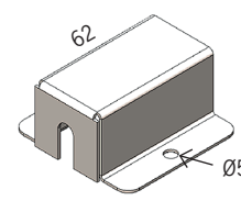
Täckande gavelfäste, rostfritt stål (tillval)
