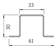
Fästbygel, rostfritt stål (standard)
