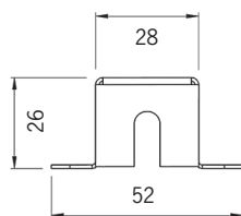
Fästbygel gavel, rostfritt stål
