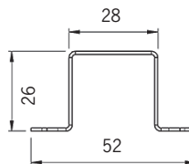
Fästbygel övergång, rostfritt stål
