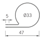
Standard: Överfångsklämma
