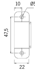
Fästbygel gavel 1025668
